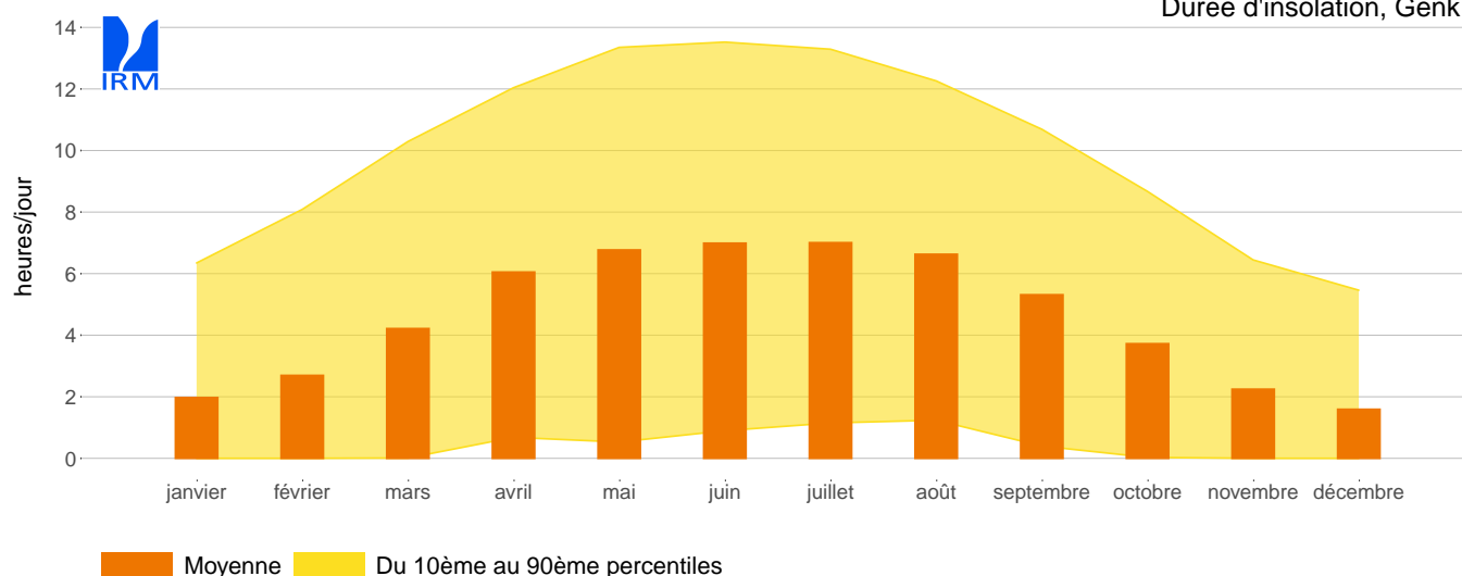
Durée d'insolation, Genk
