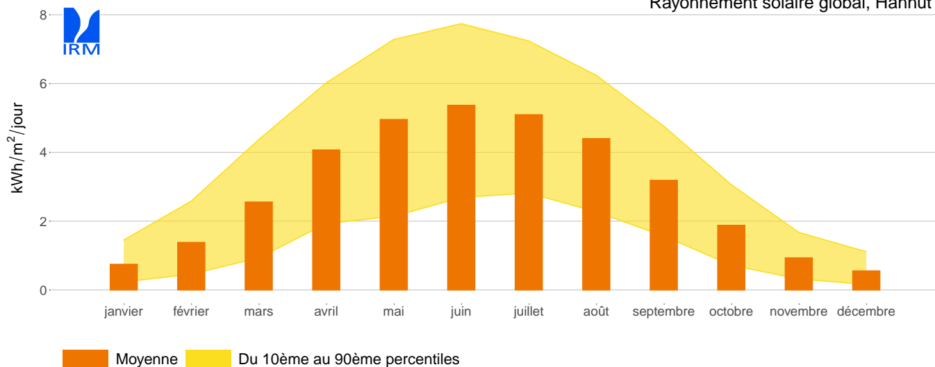
Rayonnement solaire global, Hannut
