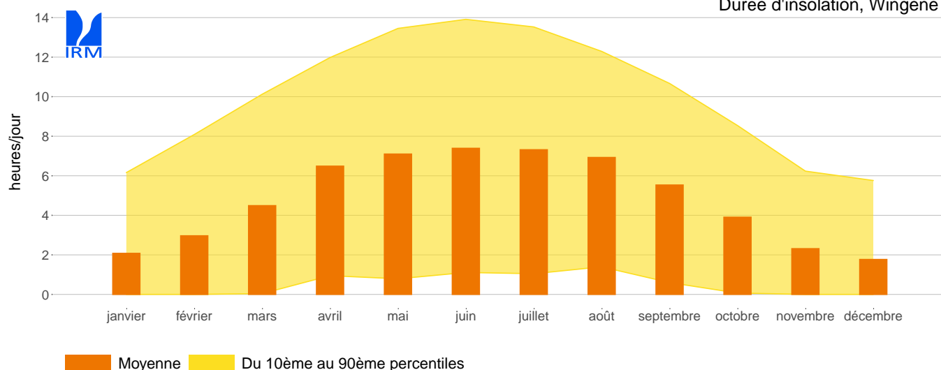
Durée d'insolation, Wingene
