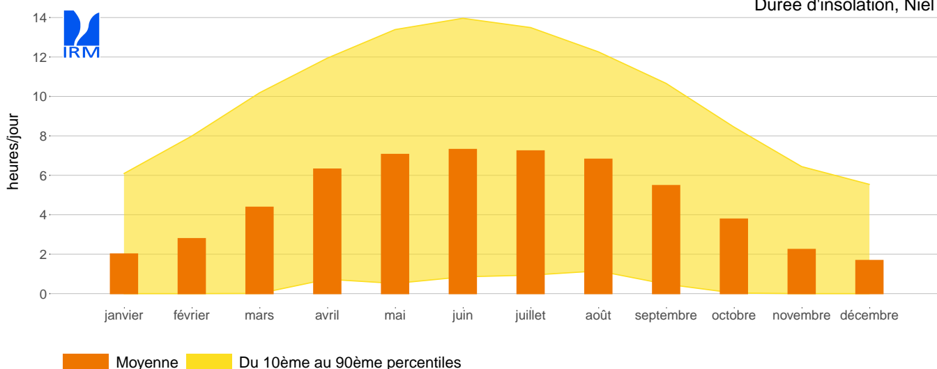
Durée d'insolation, Niel
